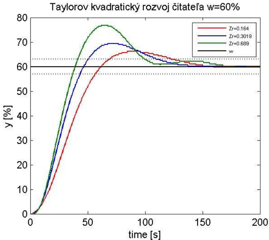
obr. Priebeh riadenia pre Taylorov kvadraticky rozvoj do čitateľa w = 60%
