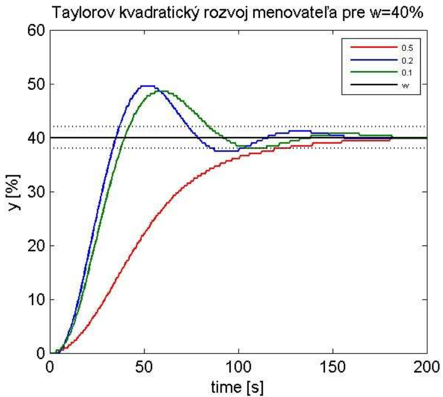
obr. 26 Priebek riadenia pre Taylorov kvadratický rozvoj do menovateľa w = 40\%
