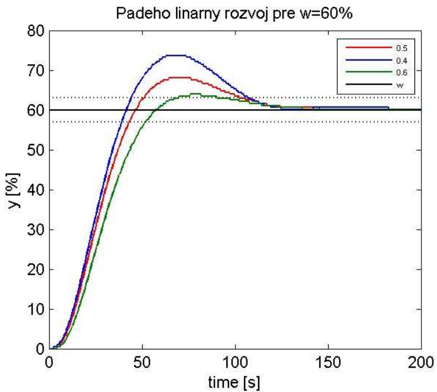
obr. 20 Priebec riadenia pre Padého lineárny rozvoj w = 60\%
