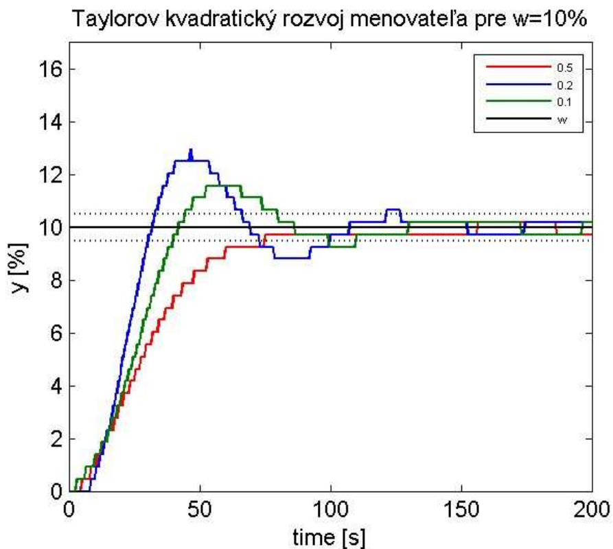
obr. 26 Priebeh riadenia pre Taylorov kvadraticky rozvoj do menovateľa w = 10\%
