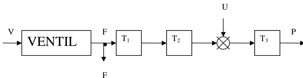
Obr. 9 bloková schéma modelu
