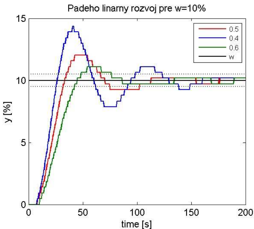
obr. 18 Priebeh riadenia pre Padého lineárny rozvoj w = 10\%
