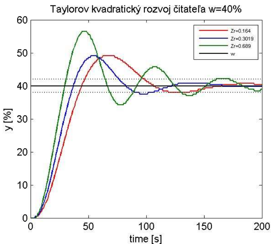
obr. 23 Priebeh riadenia pre Taylorov kvadraticky rozvoj do čitateľa w = 40\%
