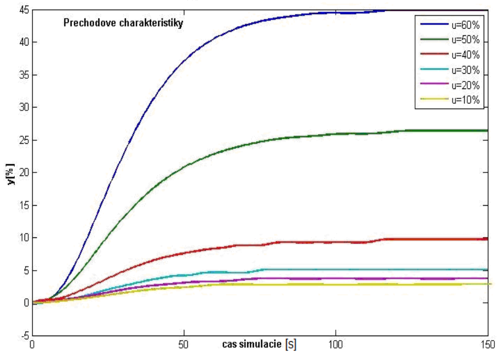
obr. 10 Zobrazenie výsledných prechodových charakteristik
