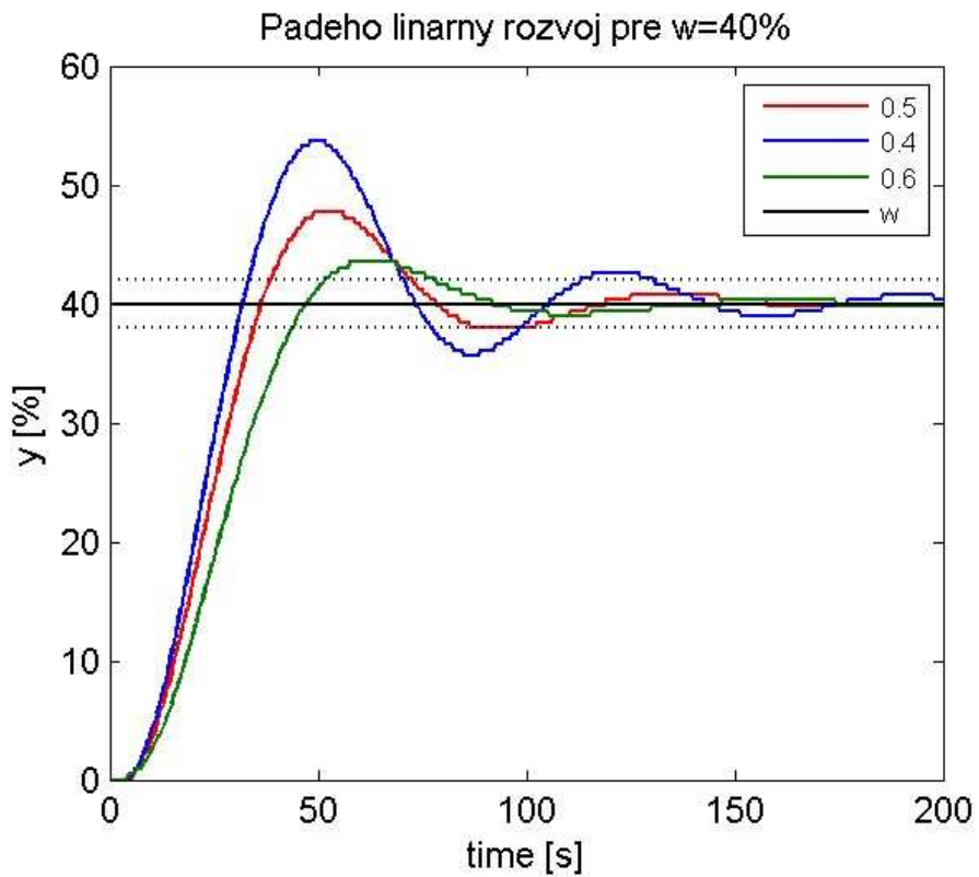
obr. 19 Priebec riadenia pre Padého lineárny rozvoj w = 40\%
